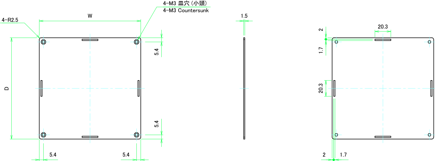
上カバー表面 / Top cover Frontside
